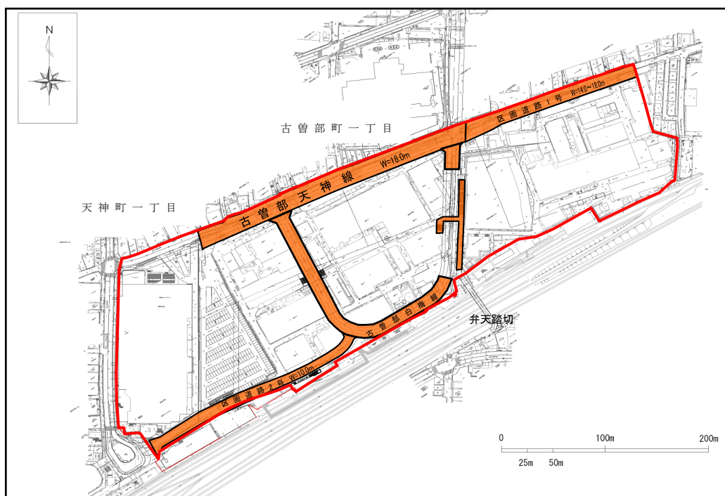
平成 21 年度整備箇所図
