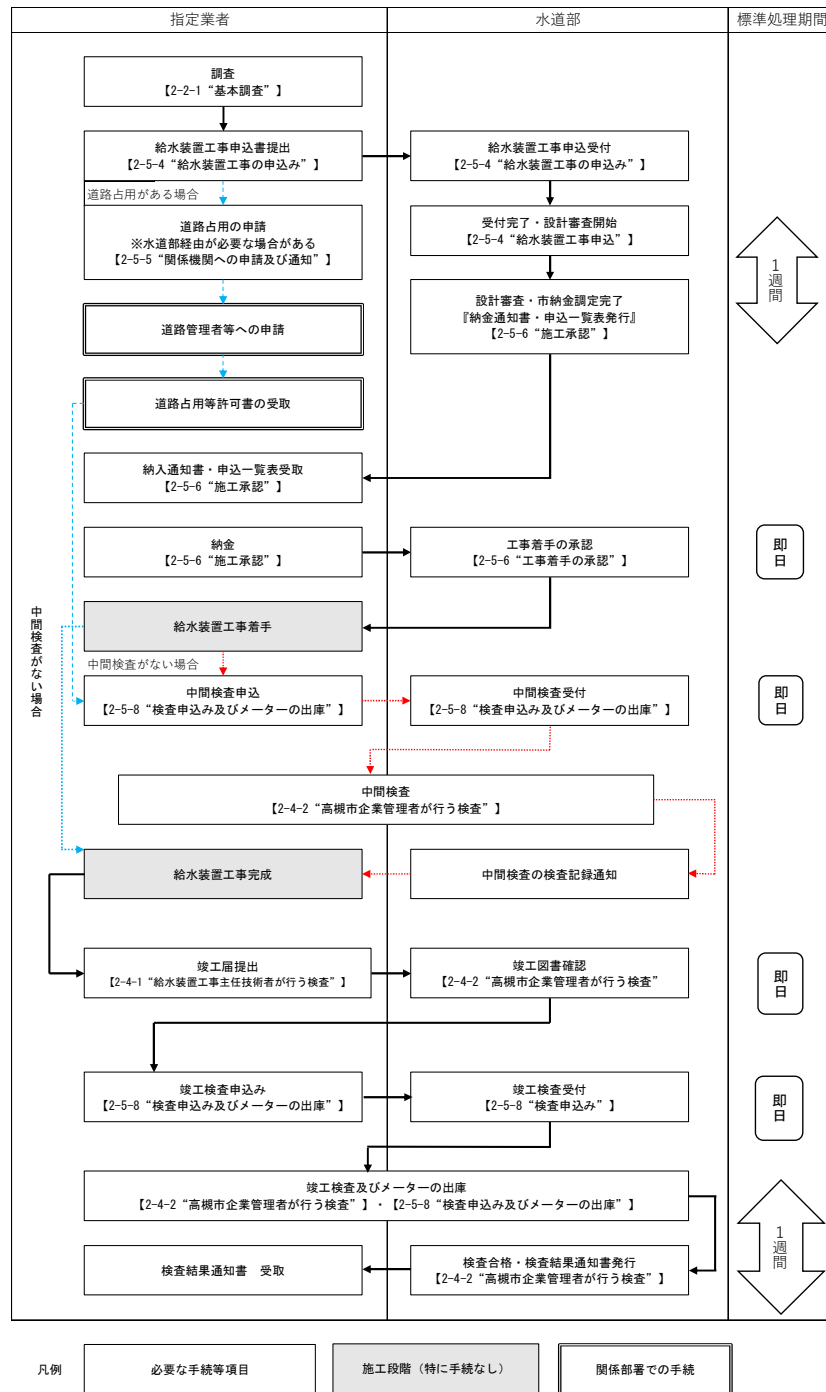
図-2.5.2.1 標準的な給水装置工事のフロー
