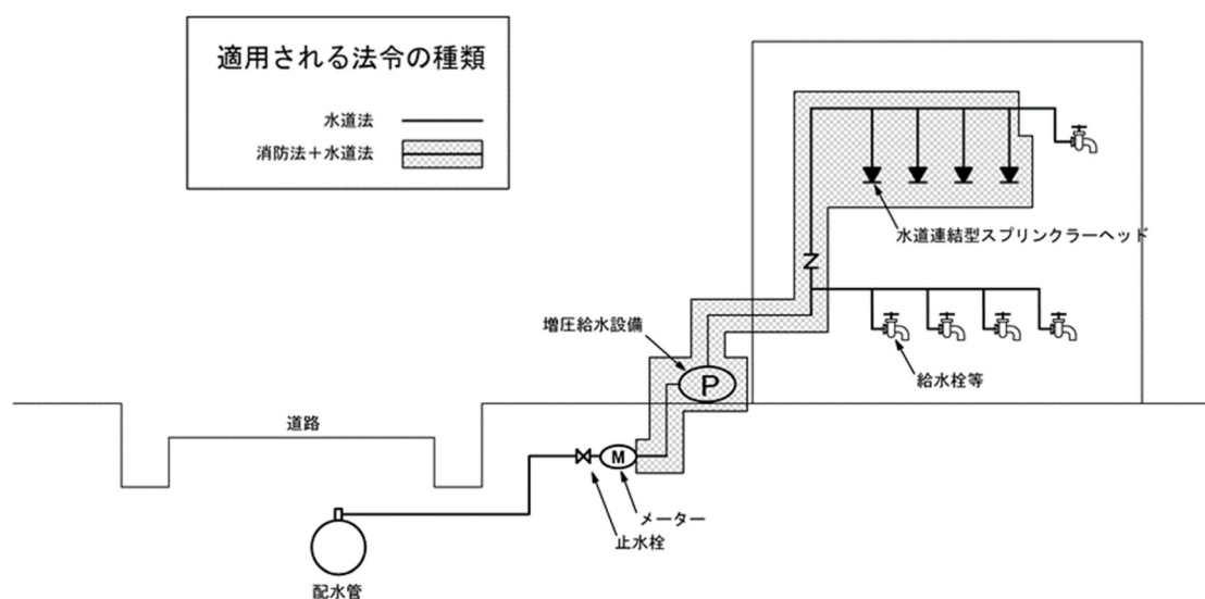
図-2.6.2.2 湿式配管（増圧）の設置例
