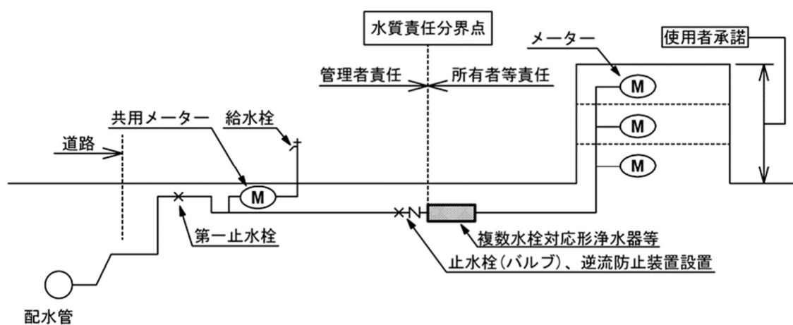
図-2.6.1.2 集合住宅における設置例
